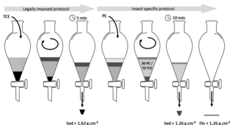
Obrázok 1. Schéma dvojitej sedimentácie PE/TCE (zdroj: EURL-AP).
